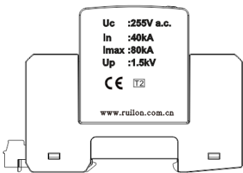
TA80-255N 标识 (Marking)
