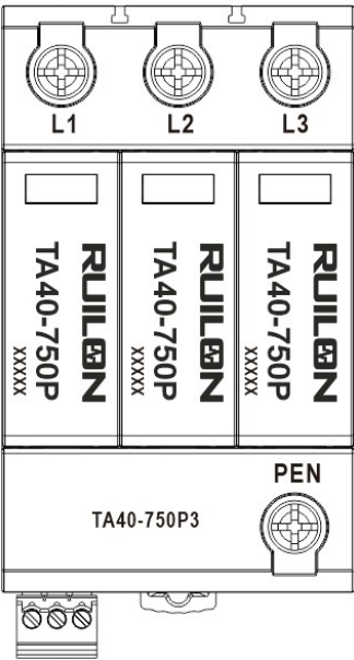
顶部标识 Top marking
